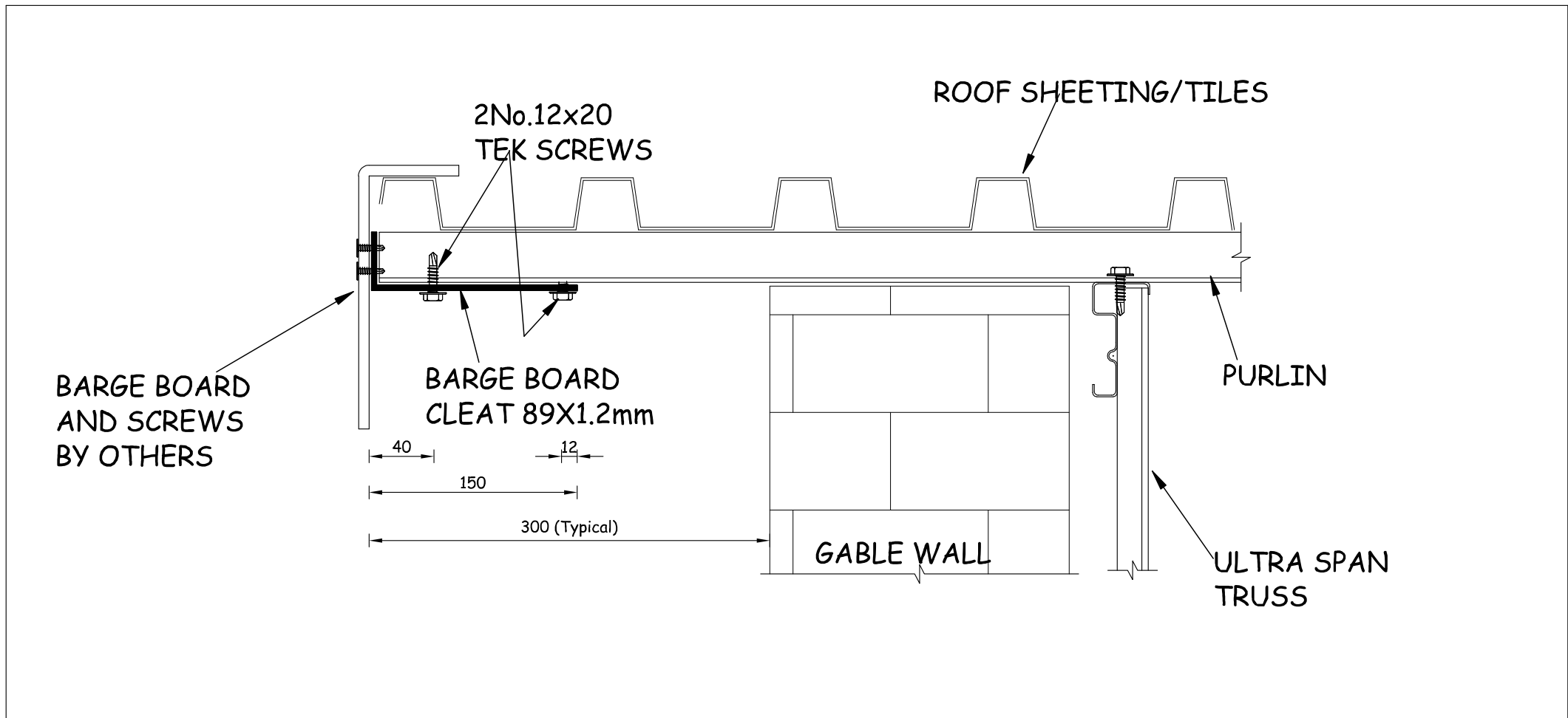
BARGEBOARD FIXING DETAIL
